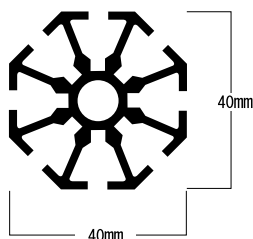
【ポール断面図】
