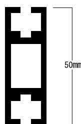
【ビーム断面図】
