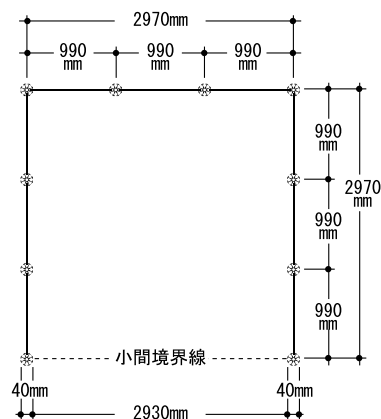
【1小間の芯々寸法】
